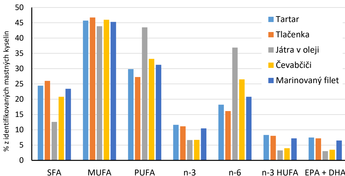
Graf 2. Zastoupení skupin mastných kyselin (v % z identifikovaných mastných kyselin) v rybích výrobcích. Data jsou průměr (n=3). SFA – nasycené mastné kyseliny; MUFA – mononenasycené mastné kyseliny; PUFA – polynenasycené mastné kyseliny; HUFA – vysoce nenasycené mastné kyseliny; EPA – kyselina eikosapentaenová; DHA – kyseliny dokosahexaenová.
